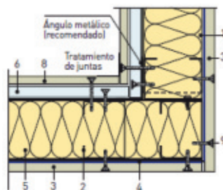
Detalle B.
