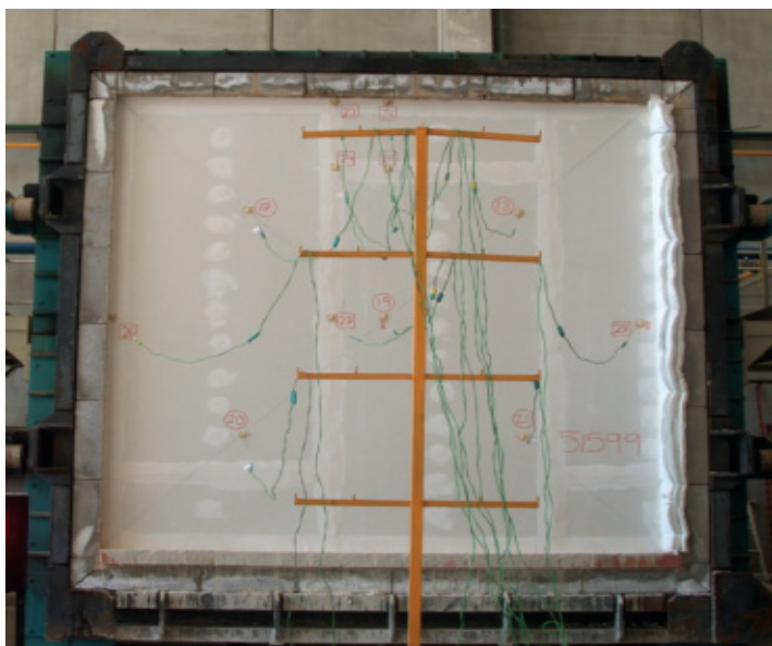
Ensayo de Resistencia al fuego en tabique. Horno de 3 x 3 m
