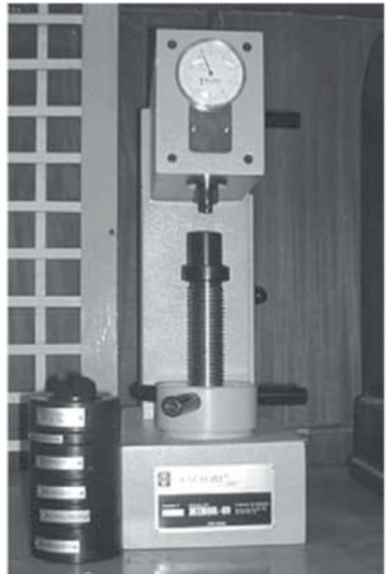
Durómetro
