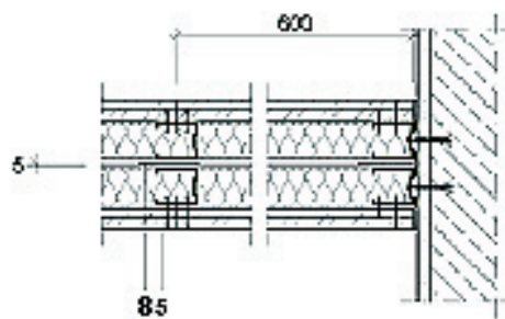
Sección horizontal
