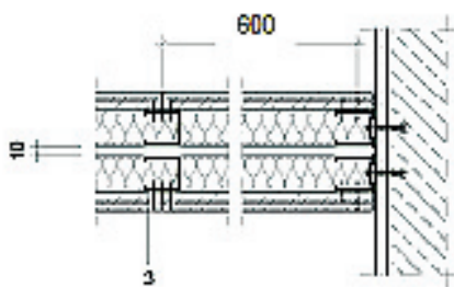
Sección horizontal
