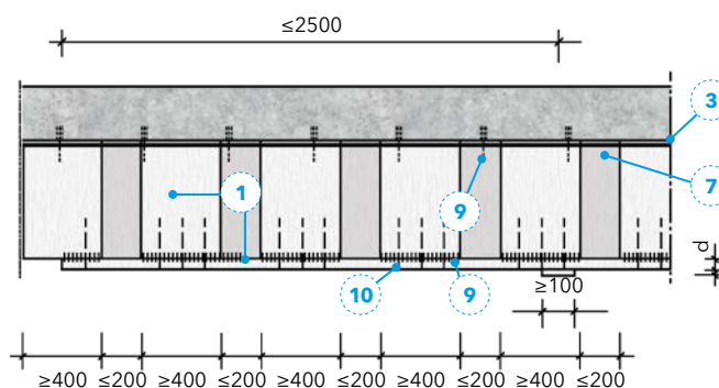
Rys. 20. Przekrój podłużny przewodu o szerokości większej niż 1250 mm i o przekroju wewnętrznym do 1,96 \text{ m}^2
