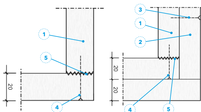
Rys. 56. Szczegół połączenia płyt w narożu
