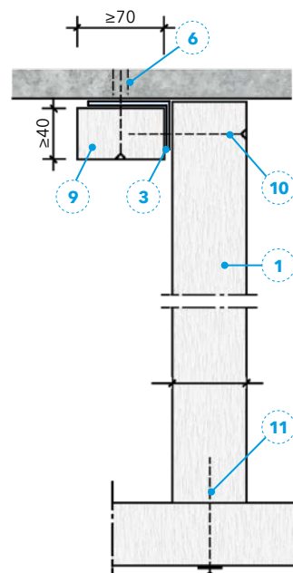
Rys. 27. Sposób połączenia usztywnienia ze stropem i dolną ścianą przewodu o szerokości większej niż 1250 mm i przekroju wewnętrznym do 1,96 m²
