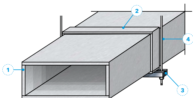
Rys. 35. Samonośny przewód wentylacji bytowej i oddymiającej PROMADUCT®-LT o przekroju wewnętrznym do 1,25 m²
