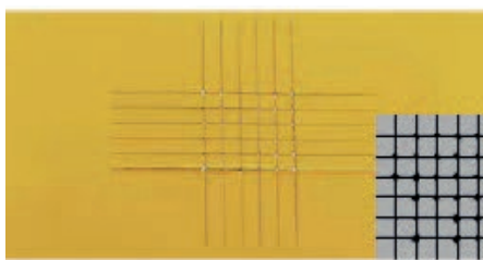
Clase ISO.: 1 / Clase ASTM.: 4 B Desprendimiento de pequeñas partes del revestimiento en las intersecciones de los cortes. No se ve significativamente afectada un área de corte mayor que 5% .
