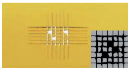
Clase ISO.: 3 / Clase ASTM.: 2 B El recubrimiento se desprende a lo largo de los bordes de los cortes, parcial o totalmente en tiras y / o se ha desprendido parcial o totalmente en diferentes partes de los cuadrados de la rejilla. Se encuentra afectada un área de corte en rejilla significativamente mayor que el 15%, pero no significativamente mayor que el 35%.
