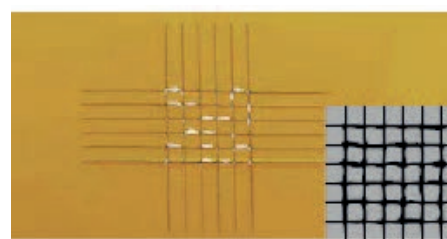
Clase ISO.: 2 / Clase ASTM.: 3 B El recubrimiento tiene desprendimientos a lo largo de los bordes y / o en las intersecciones de los cortes. Se ve afectada un área de la rejilla significativamente mayor que el 5%, pero no significativamente mayor que el 15%.
