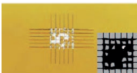
Clase ISO.: 4 / Clase ASTM.: 1 B El revestimiento se ha desprendido en los bordes de los cortes en grandes tiras, y / o algunos cuadrados se han desprendido parcial o totalmente. Se ve afectada un área de la rejilla significativamente mayor que el 35%, pero no significativamente mayor que el 65%.
