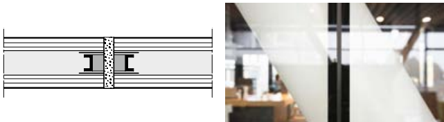
385er Konstruktionen mit Promat®-SYSTEMGLAS F1
