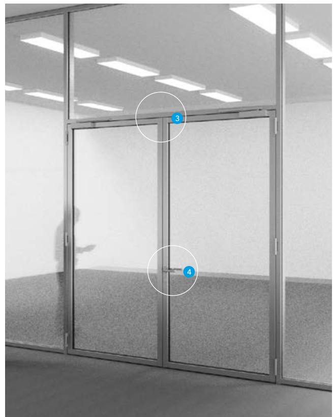
3 Die PROMAGLAS®-Systemtür F1-30 (385.36) mit schmalen Stahlhohlprofilen
