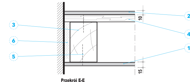
Detal E - Uszczelnienie połączenia ze ścianą
