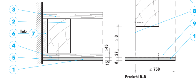
Detal C - Uszczelnienie połączenia ze ścianą
