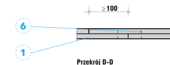
Detal G - Zabezpieczenie styków płyt
