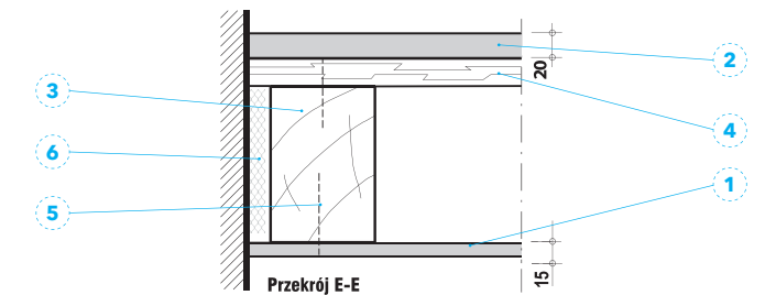
Detal E - Uszczelnienie połączenia ze ścianą
