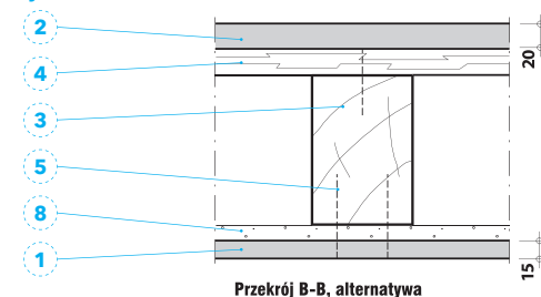
Detal C - Przekrój poprzeczny, alternatywne rozwiązanie z istniejącym tynkiem
