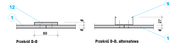
Detal H - Zabezpieczenie styków płyt
