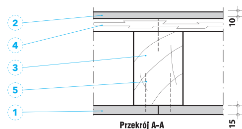
Detal B - Przekrój poprzeczny
