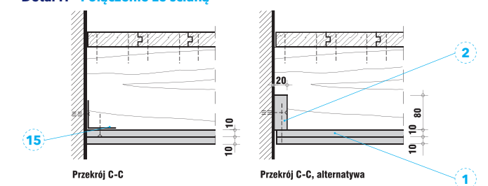
Detal H - Połączenie ze ścianą
