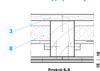
Detal D - Przekrój poprzeczny
