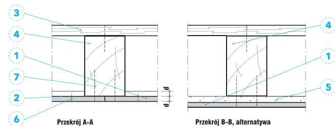
Detal B - Przekrój poprzeczny
