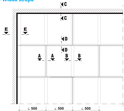
Detal A - Widok stropu
