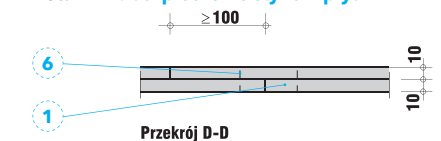
Detal I - Zabezpieczenie styków płyt
