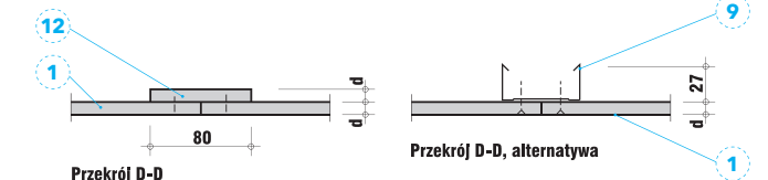
Detal H - Zabezpieczenie styków płyt
