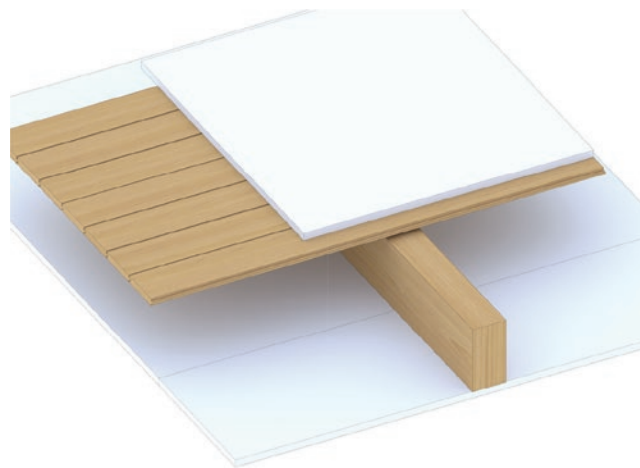
Detal A - Widok stropu
