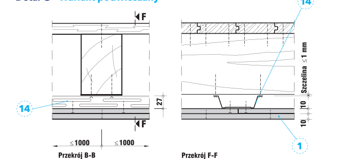
Detal G - Wariant podwieszany
