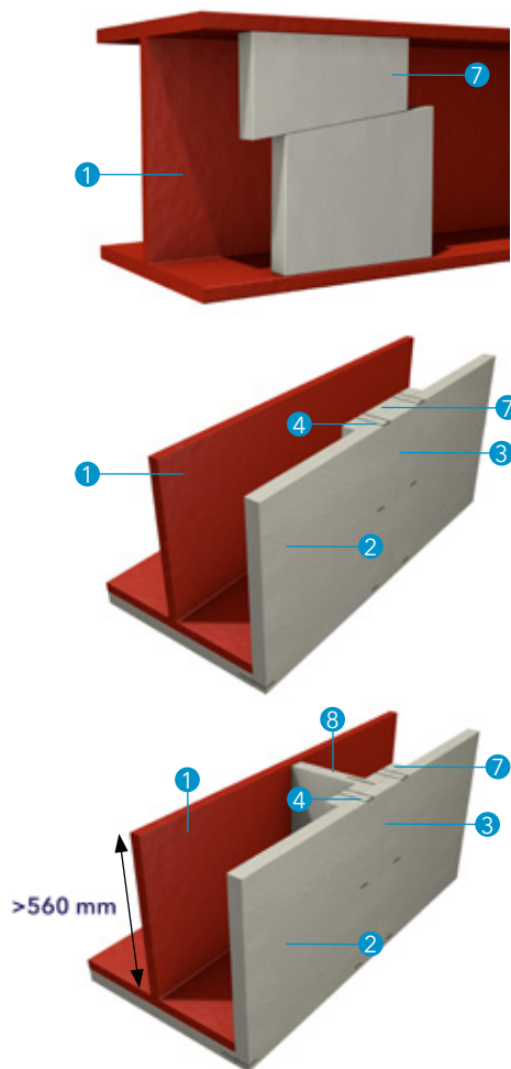
C, D és E részlet - kialakítási példa
