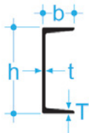
6. táblázat - UPE szelvények profiltényezői
