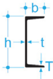
7. táblázat - UPN (UNP) szelvények profiltényezői
