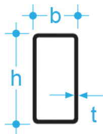
12. táblázat - Téglalap zártszelvények (RHS), EN 10210-2:2006 és EN 10219-2:2006 szerint
