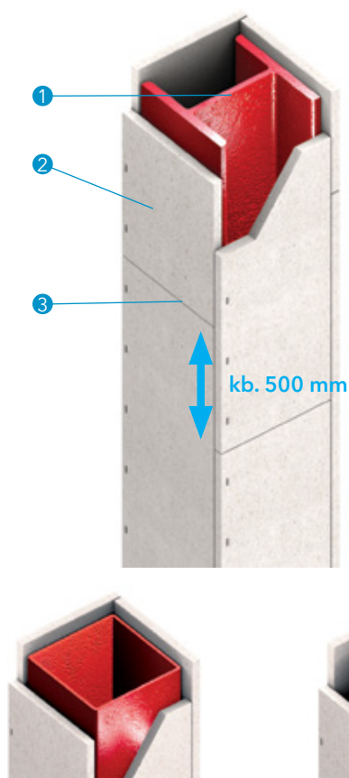
A részlet - kialakítási példa
