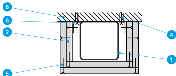
Detal B
