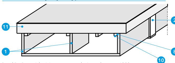
Detal B - Przewód trójścienny o szerokości większej niż 1250 mm
