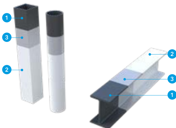
Detal A - Warstwy systemu PROMAPAIN'T SC4
