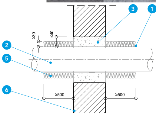
Detal A - Przejście rur stalowych i żeliwnych o średnicy powyżej 42 mm przez ściany masywne
