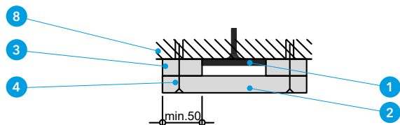
Detal A
