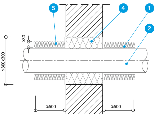
Detal C - Przejście rur stalowych i żeliwnych przez ścianę maszyną
