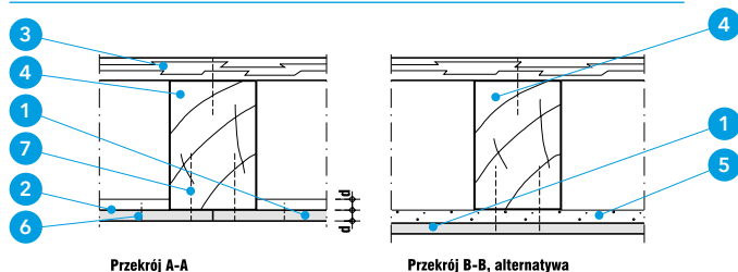
Przekrój A-A
