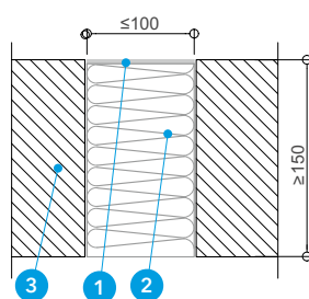
Detal E - Zabezpieczenie dylatacji w stropie
