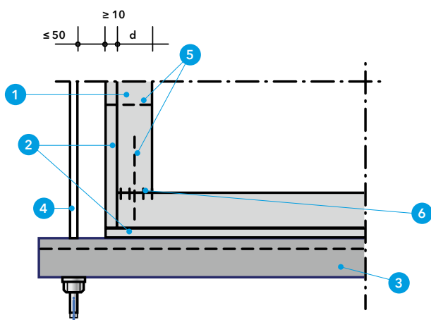
Detal C - Sposób podparcia samonośnego przewodu PROMADUCT®-LT
