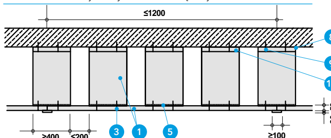
Detal C - Przekrój podłużny przewodu trójściennego
