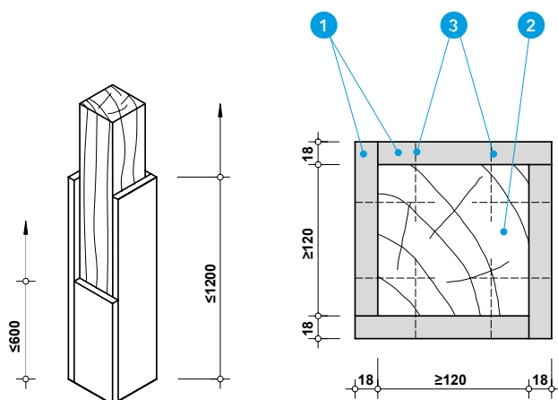
Detal A - Konstrukcja budowlana (wymiary w mm)
