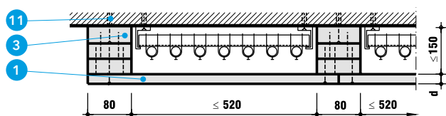
Detal I - Okładzina kabli
