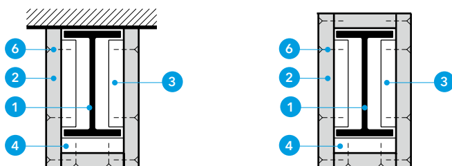
Detal B - Obudowa trójsronna i czterostronna
