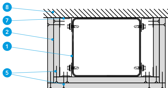
Detal C
