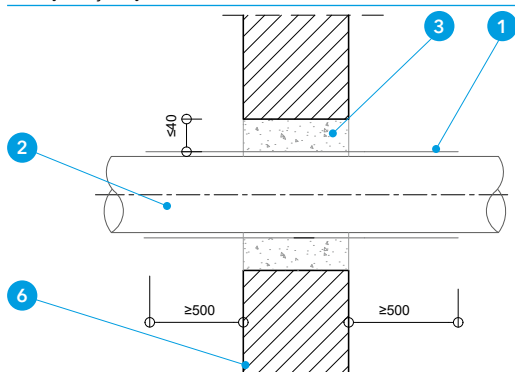
Detal B - Przejście rur stalowych i żeliwnych o średnicy do 42 mm przez ściany masywne
