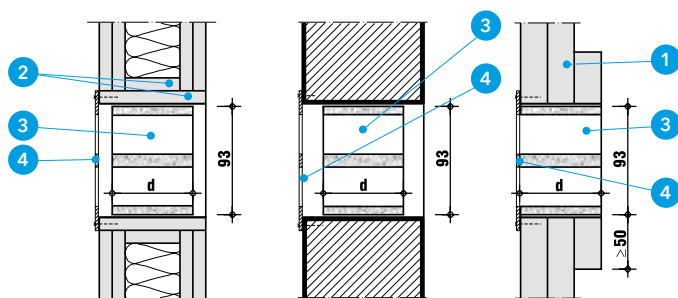
Detal D
