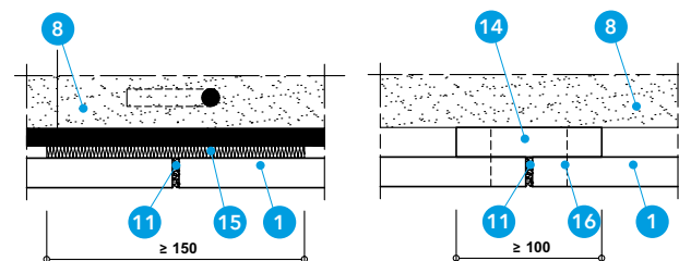
Detail H - Przekrój G-G (tylko przy płaskowniku w obszarze styków płyt) Detail H - Przekrój F-F
