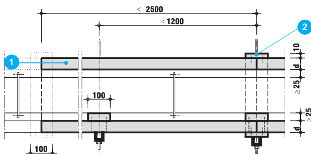
Detal B - Przekrój podłużny przez obudowę
