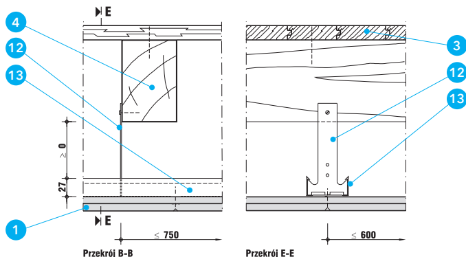
Detal F - Wariant podwieszany
