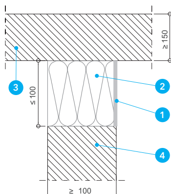
Detal B - Zabezpieczenie dylatacji pomiędzy stropem i ścianą
