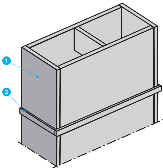
Detal A - Przewód czterościenny o szerokości większej niż 1250 mm i przekroju wewnętrznym nie większym niż 2,178 m 2 – przekrój poprzeczny
