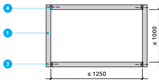
Detal B - Przewód czterościenny o przekroju wewnętrznym do 1,25 m 2
