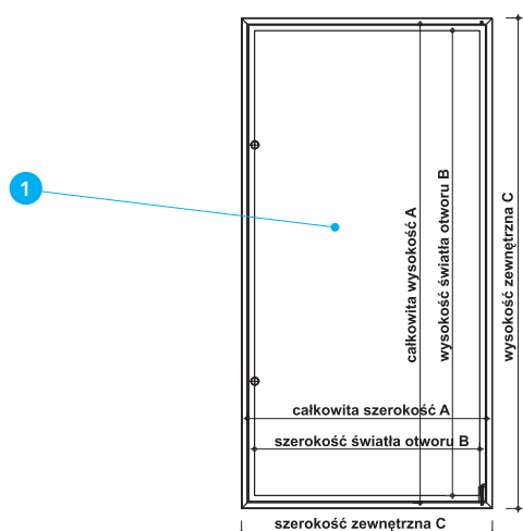
Detal A - Wymiary
