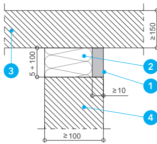
Detal F – Zabezpieczenie dylatacji w stropie pomiędzy stropem i ścianą
