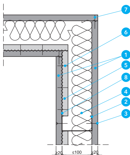
Detal B - Szczegół montażu
