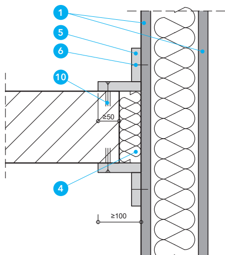
Detal E - Zabezpieczenia przejścia szachtu przez strop
