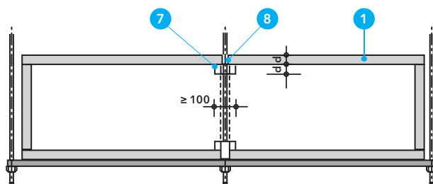
Detal F - Samonośny przewód PROMADUCT®-LT o szerokości większej niż 2000 mm i przekroju wewnętrznym nie większym niż 2,178 m 2
