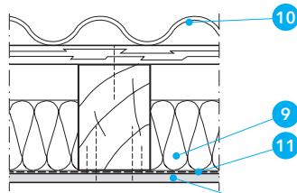
Przekrój B-B
