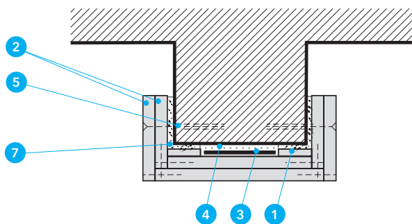
Detal B - Zabezpieczenie zbrojenia wzmacniającego, belkę
