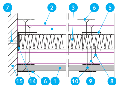
Detal C - Przekrój poprzeczny B-B
