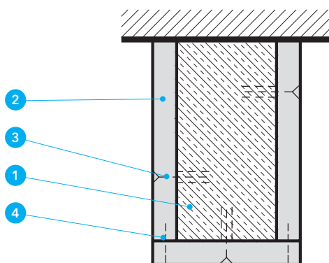
Detal A - Sposób montażu do belki
