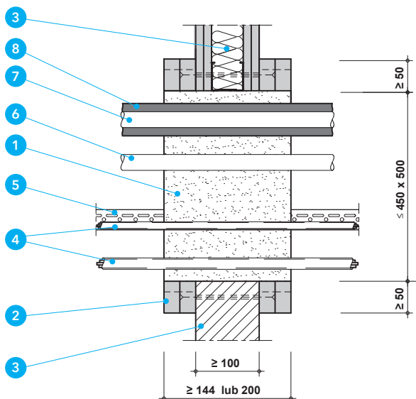
Detal A - Przejście kombinowane PROMAFOAM®-2C do kabli i rur w lekkich ścianach działowych lub ścianach masywnych
