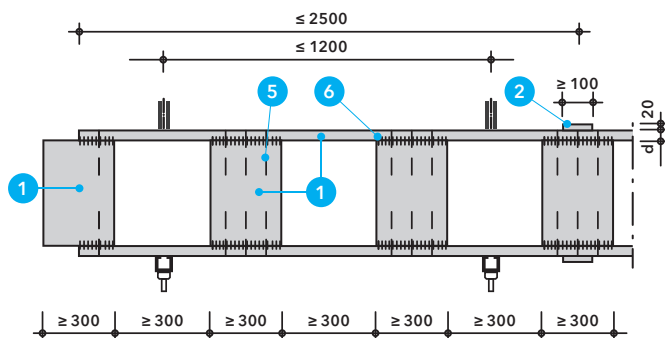
Detal E - Samonośny przewód PROMADUCT®-LT o szerokości 1251÷2000 mm i przekroju wewnętrznym nie większym niż 2,178 m 2 - przekrój podłużny
