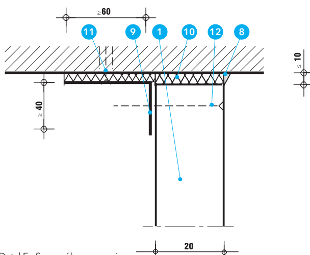
Detal E - Szczegóły mocowania
