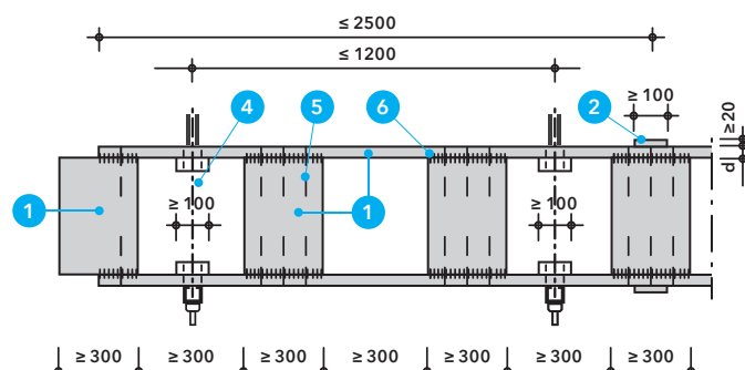
Detal G - Samonośny przewód PROMADUCT®-LT o szerokości większej niż 2000 mm i przekroju wewnętrznym nie większym niż 2,178 m 2 - przekrój podłużny
