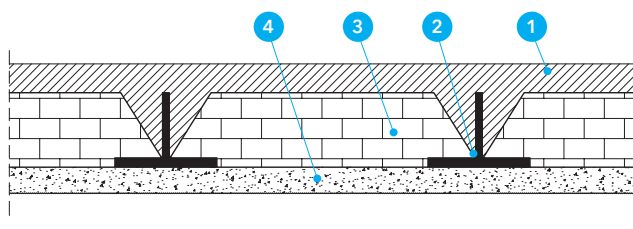
Detal A – strop z belkami stalowymi i wypełnieniem z pustaków ceramicznych
