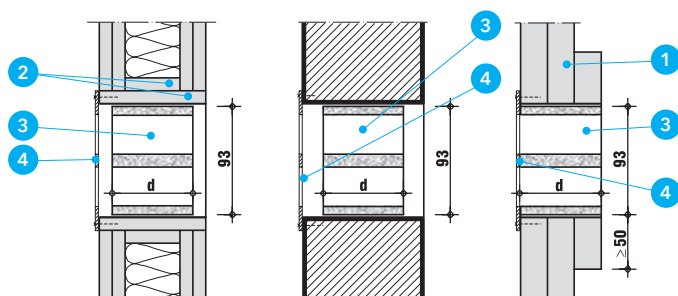
Detal D
