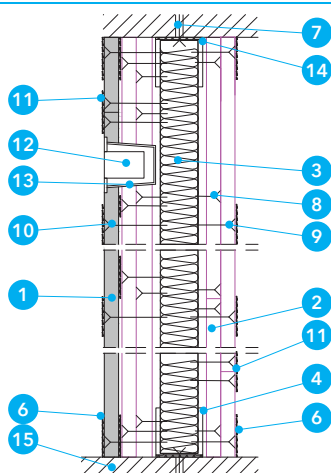
Detal B - Pionowy przekrój A-A
