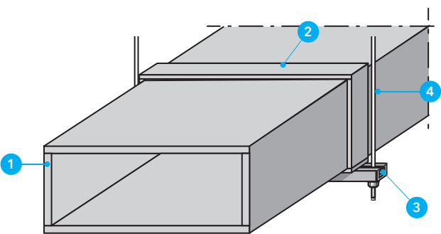
Detal A - Samonośny przewód wentylacji bytowej i oddymiającej PROMADUCT®-LT o przekroju wewnętrznym do 1,25 m 2
