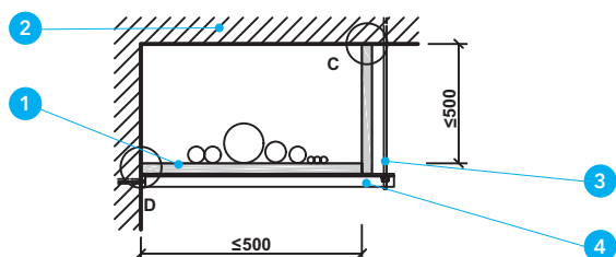
Detal A - Konfiguracje kanałów instalacyjnych
