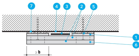
Detal A - Zabezpieczenie zbrojenia wzmacniającego, klejonego od dołu stropu
