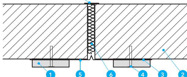
Detal B - Uszczelnienie dylatacji za pomocą masy PROMASEAL®-A Spray
