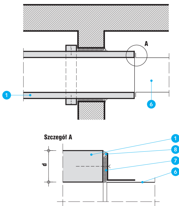
Detal E - Połączenie z kanałem z blachy stalowej
