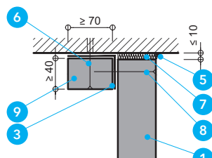
Detal B - Metoda mocowania płyt do ściany betonowej
