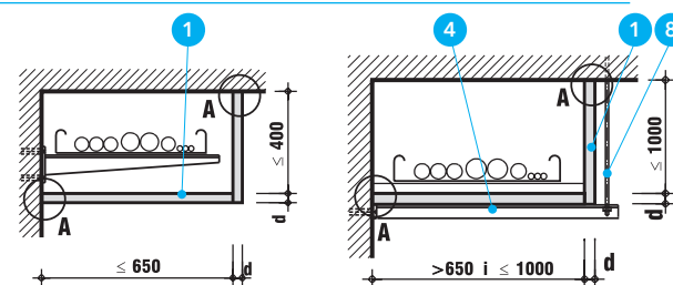
Detal F - Kanał dwustronny
