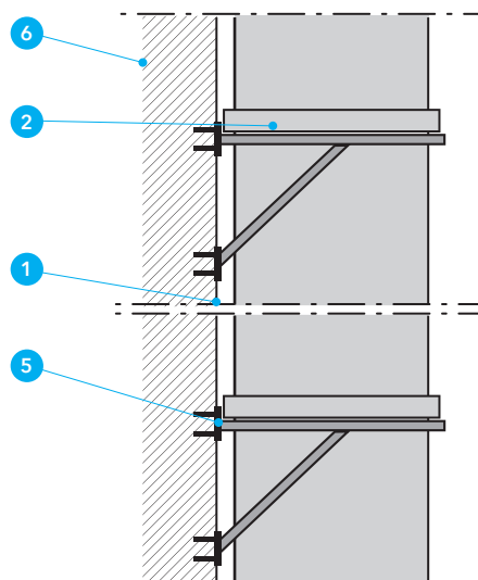
Detal D - Konstrukcja wsporcza przewodu
