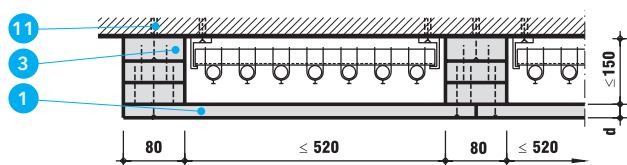
Detal I - Okładzina kabli
