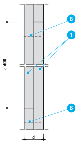
Przekrój B-B
