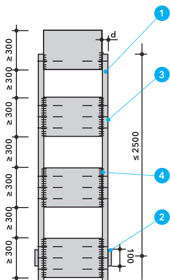
Detal C - Przewód czterościenny o szerokości większej niż 1250 mm i przekroju wewnętrznym nie większym niż 2,178 m 2 - przekrój podłużny
