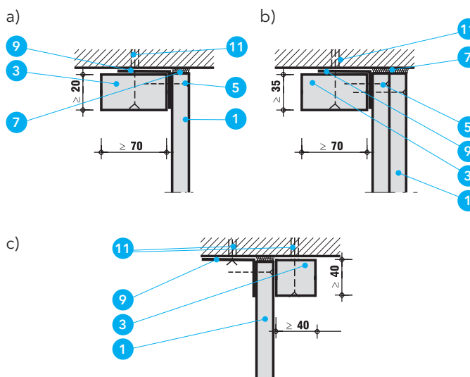
Detal G - Szczegół połączenia kanału ze stropem lub ścianą
