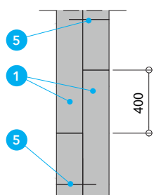
Detal C - Przekrój pionowy
