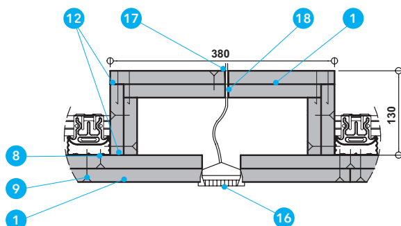
Detal D - Montaż oświetlenia
