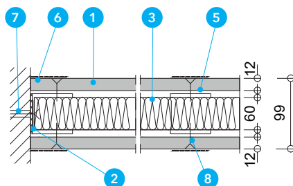
Detal C – Przekrój poprzeczny B-B
