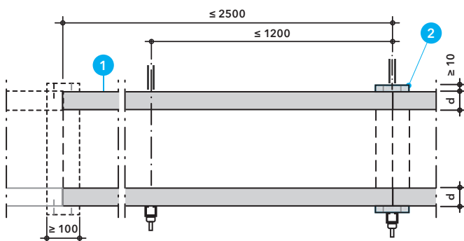
Detal B - Samonośny przewód PROMADUCT®-LT o szerokości nie większej niż 1250 mm i przekroju wewnętrznym nie większym niż 1,25 m 2 - przekrój podłużny
