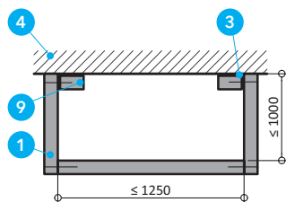
Detal A - Przewód w konfiguracji trójściennej
