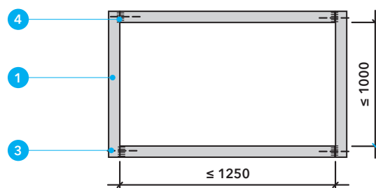
Detal B - Przewód czterosienny o przekroju wewnętrznym do 1,25 m 2
