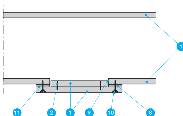
Detal C - Rewizja w przewodzie PROMADUCT®-LT
