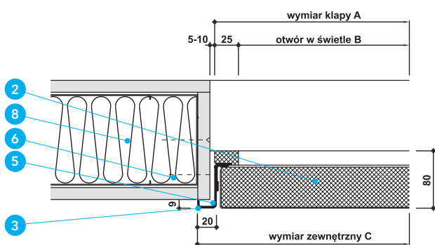
Detal B - Sposób montażu w ścianie lekkiej
