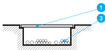
Detal C - Jednostronny kanał kablowy
