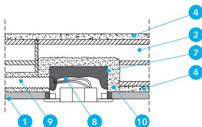
Detal C - Montaż puszki elektrycznej
