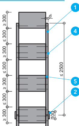
Detal C - Przekrój podłużny przewodu czterościennego
