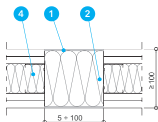
Detal B – Zabezpieczenie dwustronne dylatacji w ścianie
