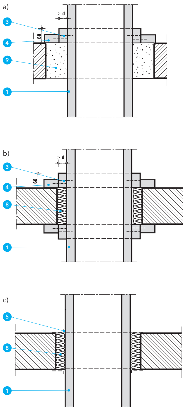
Detal C - Przejście przewodów przez strop
