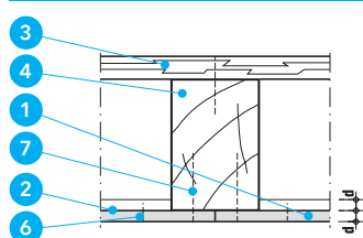
Przekrój A-A
