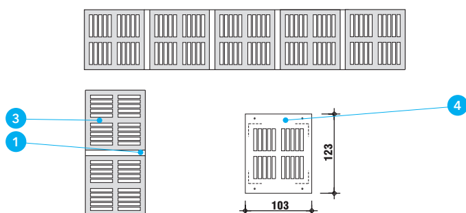
Detal A
