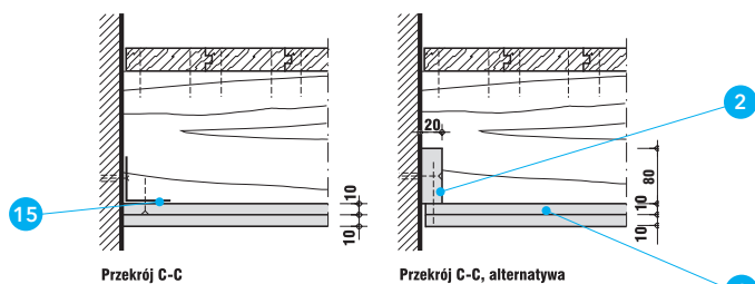
Detail H - Połączenie ze ścianą
