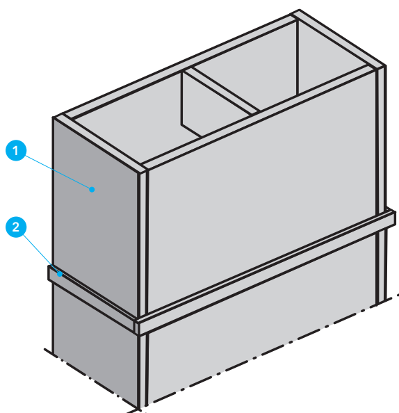
Detal A - Przewód czterosienny o szerokości większej niż 1250 mm i przekroju wewnętrznym nie większym niż 2,178 m 2 – przekrój poprzeczny
