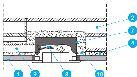
Detal C – Montaż puszek elektrycznej
