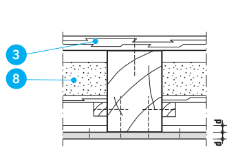
Przekrój B-B
