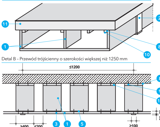
Detal C - Przekrój podłużny przewodu trójściennego
