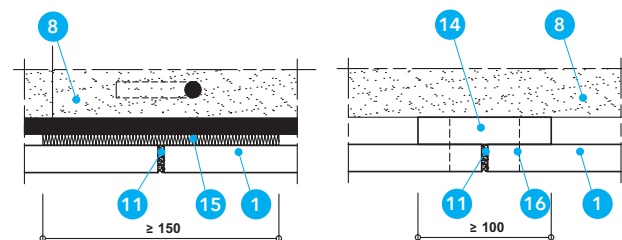
Detail H - Przekrój G-G (tylko przy płaskownicy w obszarze styków płyt) i Detail H - Przekrój F-F
