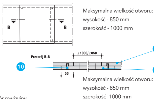
Detal D - Otwór rewizyjny
