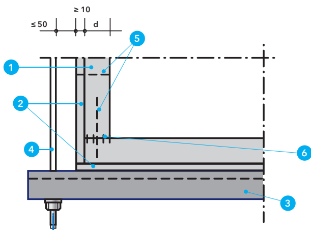
Detal C - Sposób podparcia samonośnego przewodu PROMADUCT®-LT
