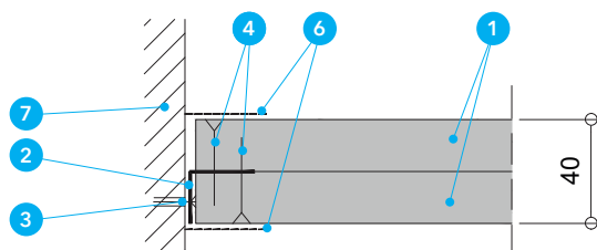
Detal B - Połączenie z innymi przegrodami budowlanymi lub konstrukcją budynku
