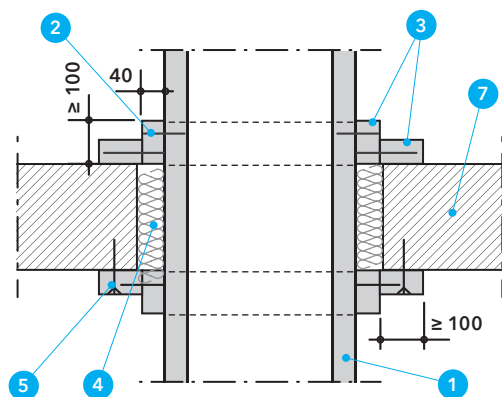
Detal B - Przejście przez strop przewodu samonośnego PROMADUCT®-LT.
