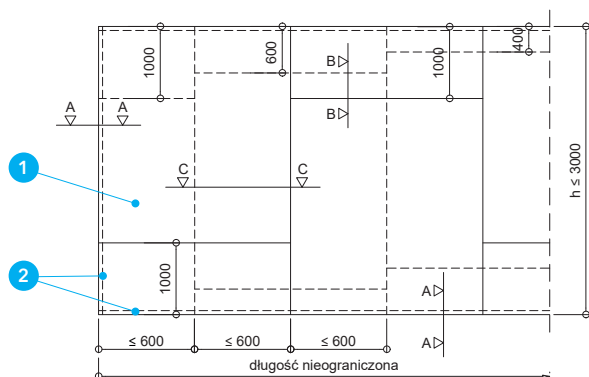
Detal A - Widok ściany
