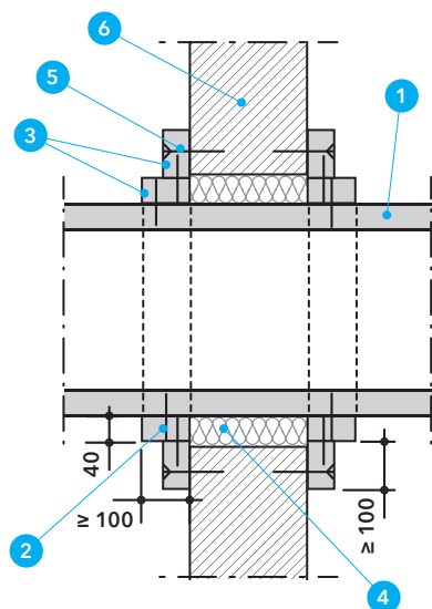
Detal A - Przejście przez ścianę przewodu samonośnego PROMADUCT®-LT.
