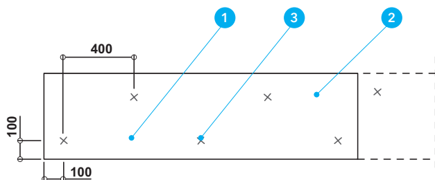
Detal B - Widok mocowania płyt do boku belki lub słupa
