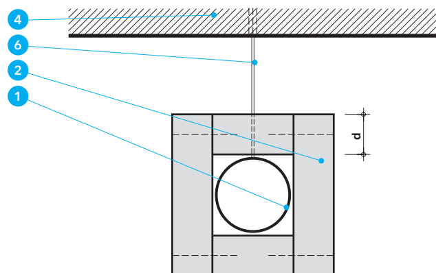
Detal B - Czterostronna okładzina przewodu oraz zawieszisko
