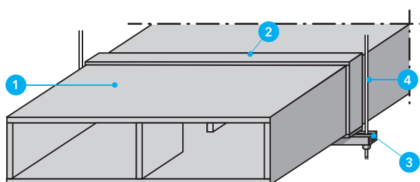
Detal D - Samonośny przewód PROMADUCT®-LT o szerokości 1251÷2000 mm
