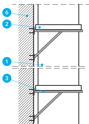
Detal B – Konstrukcja wsporcza przewodu
