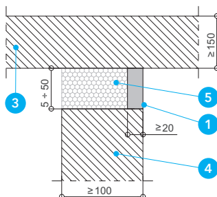
Detal D – Zabezpieczenie dylatacji wypełnionej materiałem palnym pomiędzy stropem i ścianą
