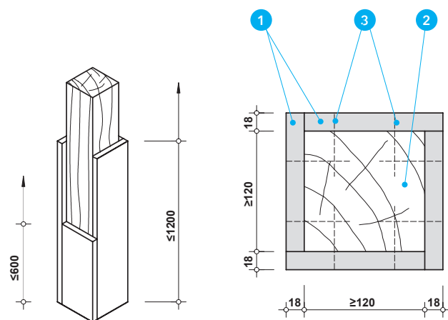
Detal A - Konstrukcja budowlana (wymiary w mm)
