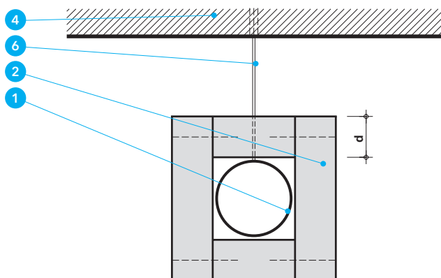
Detal B - Czerostronna okładzina przewodu oraz zawiesie
