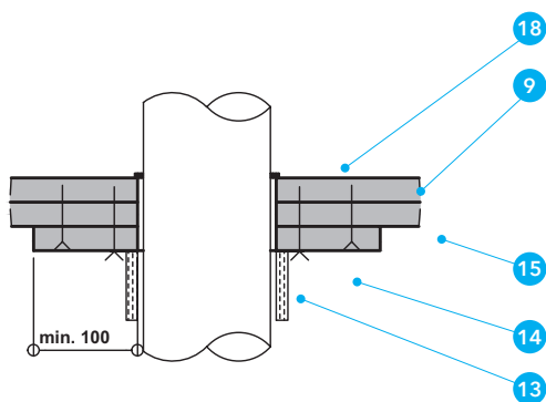
Detal C - Przejście rur palnych
