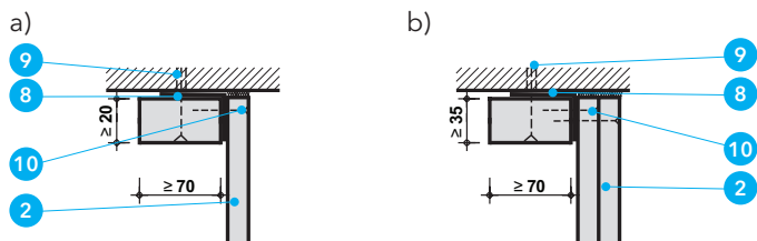
Detal C - Kanały dwustronne i trójstronne
