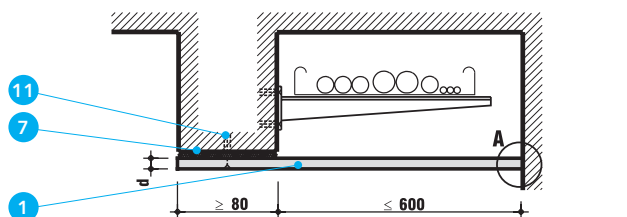
Detal H - Okładzina jednostronna
