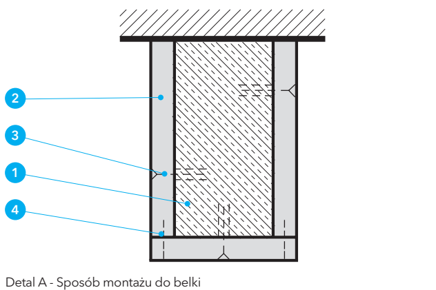
Detal A - Sposób montażu do belki
