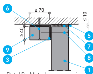
Detal B - Metoda mocowania płyt do ściany betonowej
