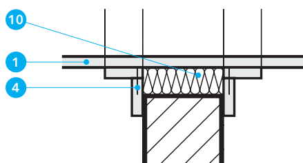
Detal G - Przejście przewodu przez przegrodę
