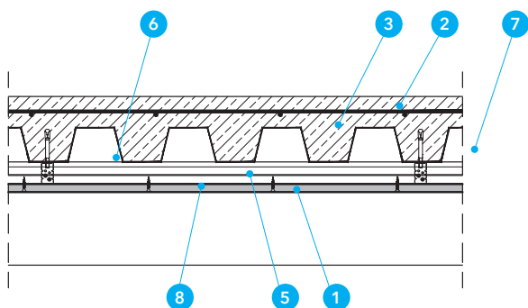
Detal B - Przekrój podłużny
