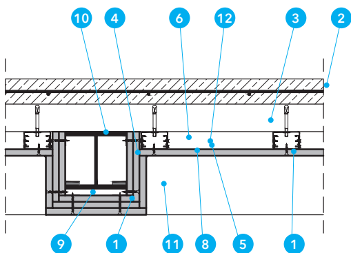
Detal A - Przekrój podłużny
