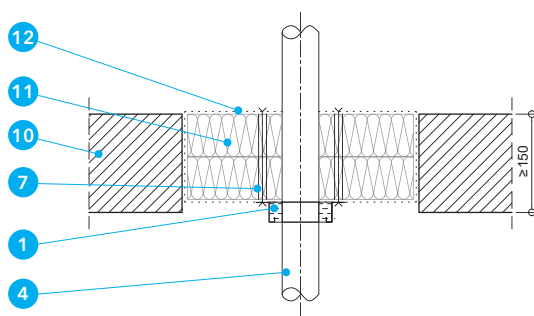
Detal D - Montaż kołnierzy pod stropem z uszczelnieniem wełną i masą ogniochronną
