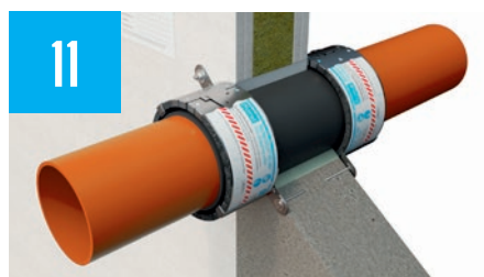
PRZEJŚCIA INSTALACYJNE 212
