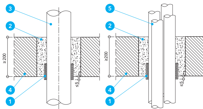
Detal C - Przejście przez strop rur z tworzywa sztucznego
