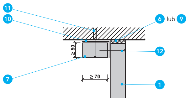
Detal C – Mocowanie kanałów dwu- i trójsięnnych do stropu
