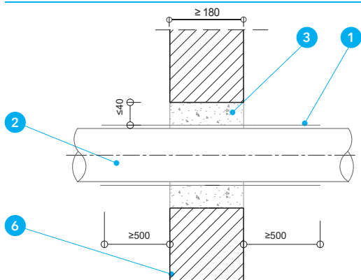
Detal B - Przejście rur stalowych i żeliwnych o średnicy do 42 mm przez ścianę masywną
