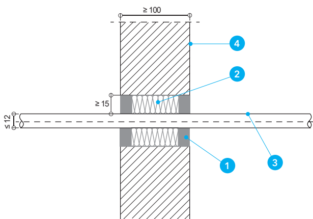
Detal A - Przejście węża pneumatycznego poliuretanowego przez ścianę
