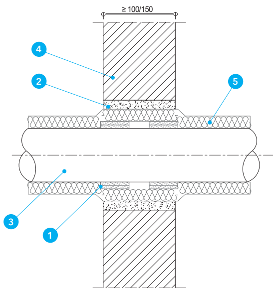
Detal A - Przejście rur z tworzywa sztucznego w izolacji z wełny skalnej przez ścianę
