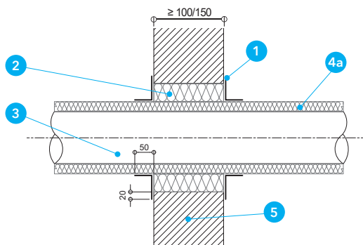
Detal A - Przejście rur stalowych przez ścianę o średnicy maks. 108 mm
