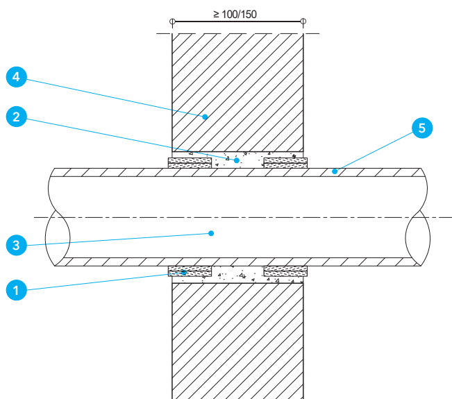
Detal A - Przejście rury stalowej w izolacji palnej przez ścianę
