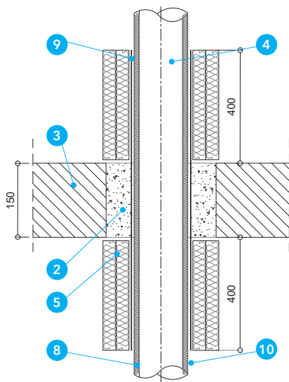
Detal B - Rura stalowa z izolacją z wełny mineralnej i płaszczem stalowym
