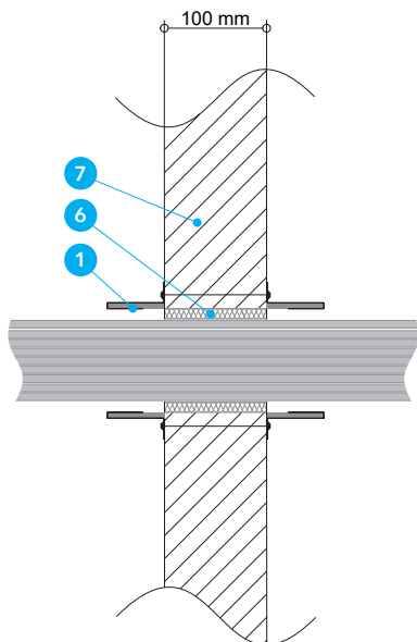
Detal D - Przejście kablowe w ścianie masywnej przy ścianie
