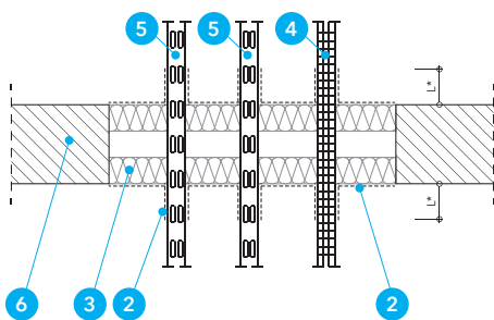
Detal C - Przejście przez strop
