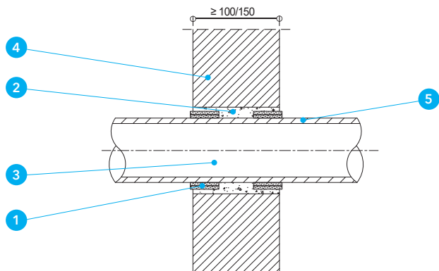
Detal A - Przejście rur z tworzywa sztucznego w izolacji palnej przez ścianę
