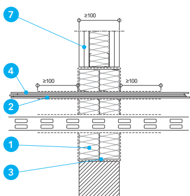
Detal A - Przejście przez ścianę gr. min. 100 mm lub strop masywny min. 150
