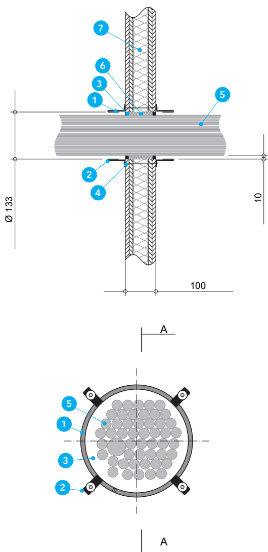
Detal A - Przejście kablowe w ścianie lekkiej lub masywnej
