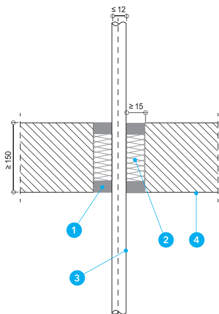
Detal B - Przejście węża pneumatycznego poliuretanowego przez strop
