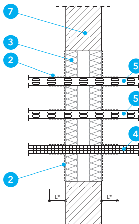
Detal B - Przejście przez ścianę gr. min. 150 mm
