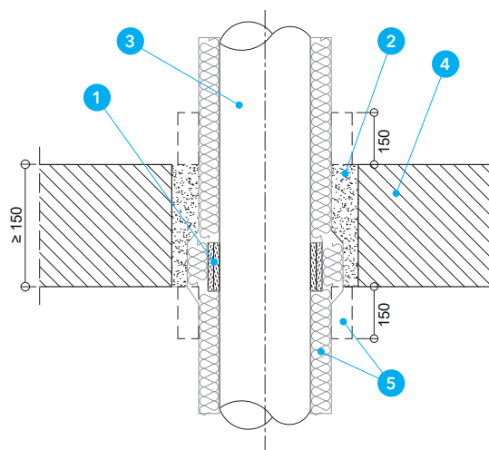
Detal B - Przejście rur z tworzywa sztucznego w izolacji z wełny skalnej przez strop
