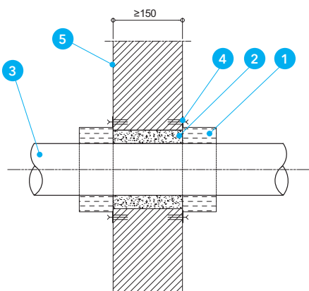
Detal A - Montaż kołnierza na ścianie
