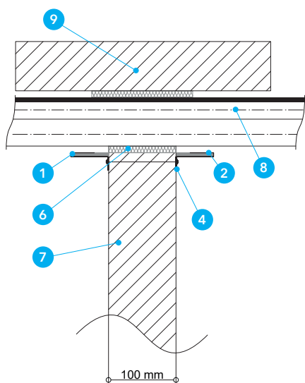
Detal C - Przejście kablowe w ścianie masywnej pod stropem
