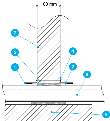
Detal B - Przejście kablowe w ścianie masywnej na stropie
