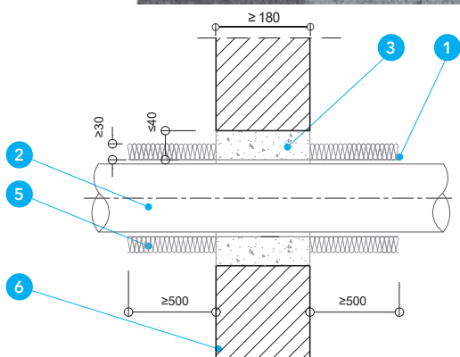
Detal A - Przejście rur stalowych i żeliwnych o średnicy powyżej 42 mm przez ścianę masywną
