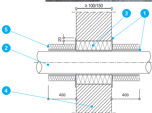
Detal A - Przejście rur aluminiowych przez ścianę
