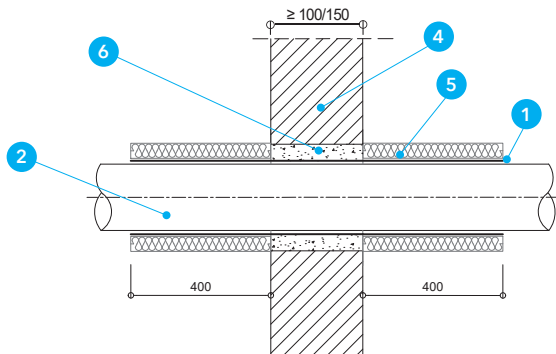
Detal B - Przejście rur miedzianych przez ścianę
