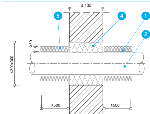
Detal C - Przejście rur stalowych i żeliwnych przez ścianę masywną
