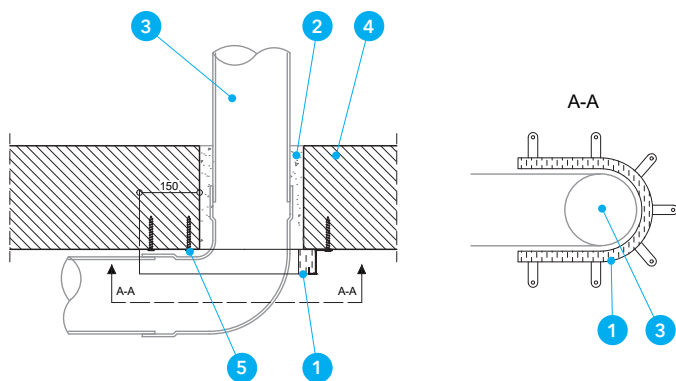
Detal A - Przejście rury z tworzywa sztucznego przez strop
