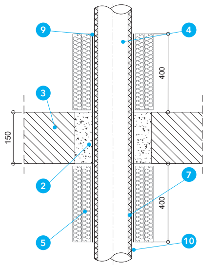
Detal C – Rura stalowa z izolacją z PUR i płaszczem stalowym
