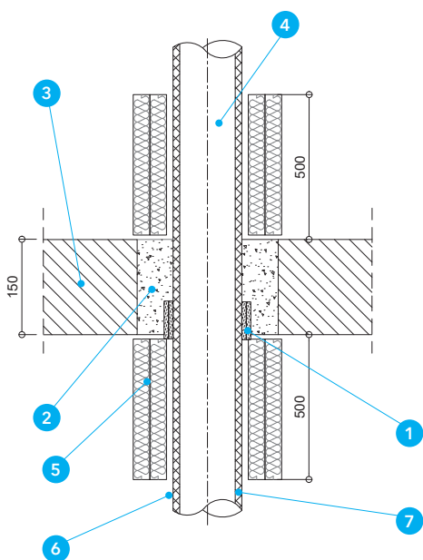
Detal A - Rura stalowa z izolacją PUR i płaszczem PE-HD
