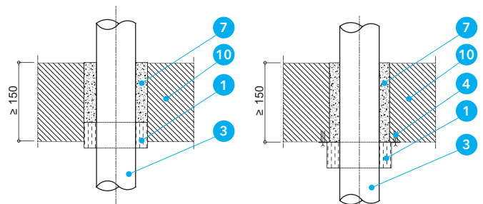
Detal C - Montaż kołnierza wewnątrz stropu
