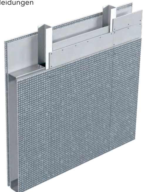
DURASTEEL® Verbund-Barrieresystem (E 240 – EI 180) mit hervorragenden Schallschutzeigenschaften.
