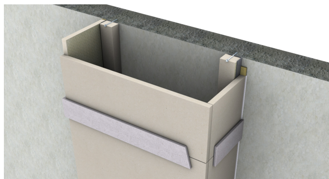
DETTAGLIO W - COLLEGAMENTO DI SPIGOLO
