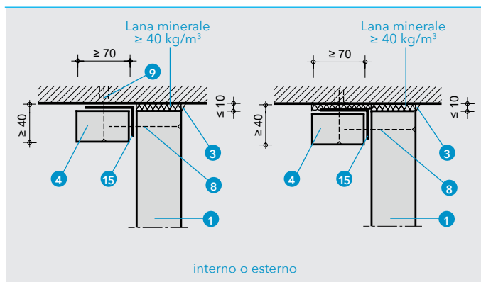
DETTAGLIO Y - SEZIONE LONGITUDINALE
