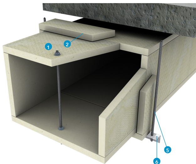
DETTAGLIO A - SEZIONE TRASVERSALE
