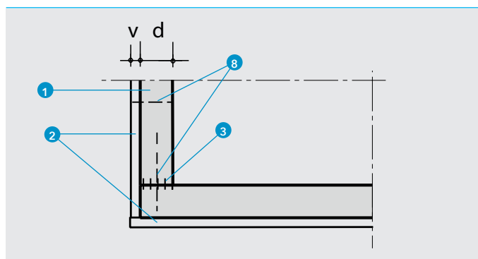
DETTAGLIO X - COLLEGAMENTO ALLA PARETE - SEZIONE TRASVERSALE
