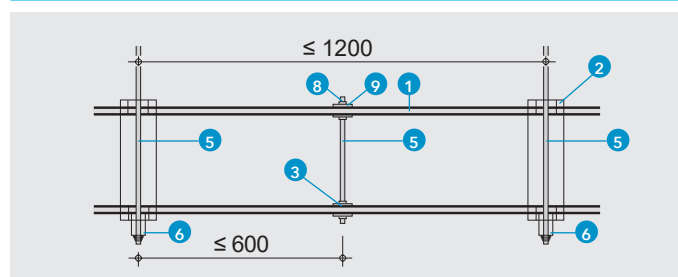
DETTAGLIO B - SEZIONE LONGITUDINALE
