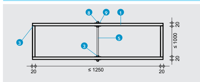
DETTAGLIO A - SEZIONE TRASVERSALE
