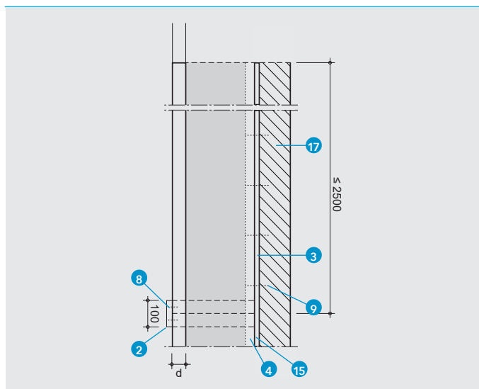
DETTAGLIO Y - SEZIONE LONGITUDINALE
